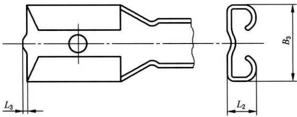
插套尺寸 mm
