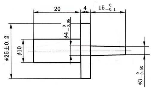
图 13 探针
