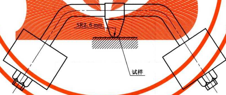
图 12 球压试验器
