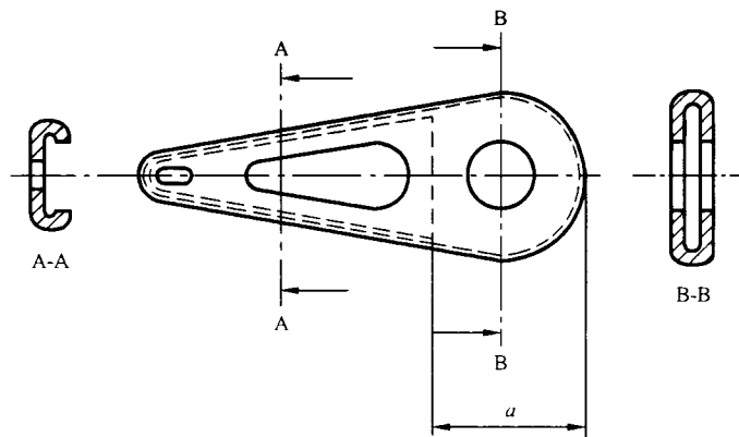
图 6 链罩
